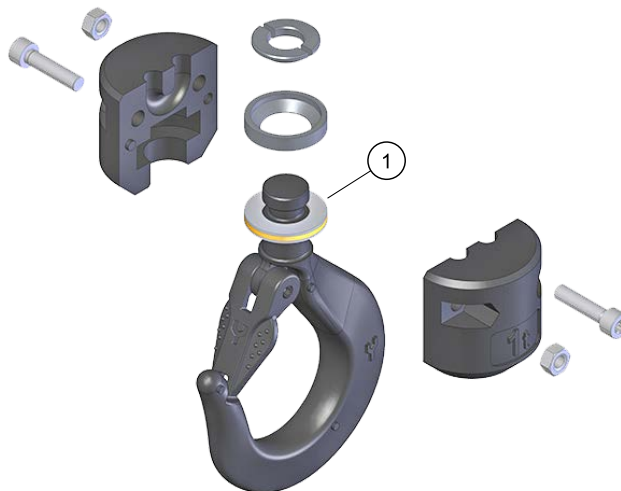
1 Palier de butée
