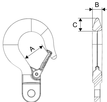
Figura 6. Critérios de remoção de ganchos
