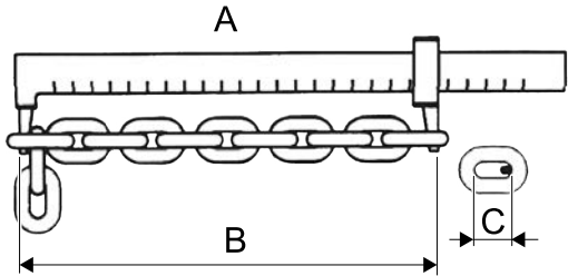
Figura 9. Medição do desgaste da corrente de carga
