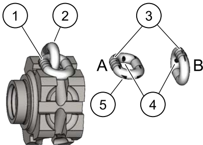
Figura 7. Áreas de desgaste de la cadena
