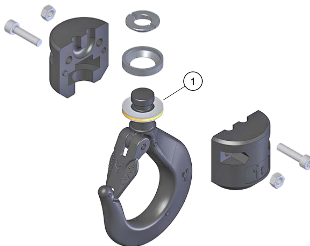
1 Rolamento axial
