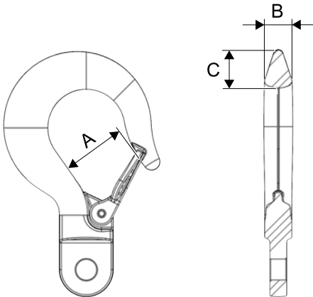
Figure 6. Critères d'enlèvement des crochets
