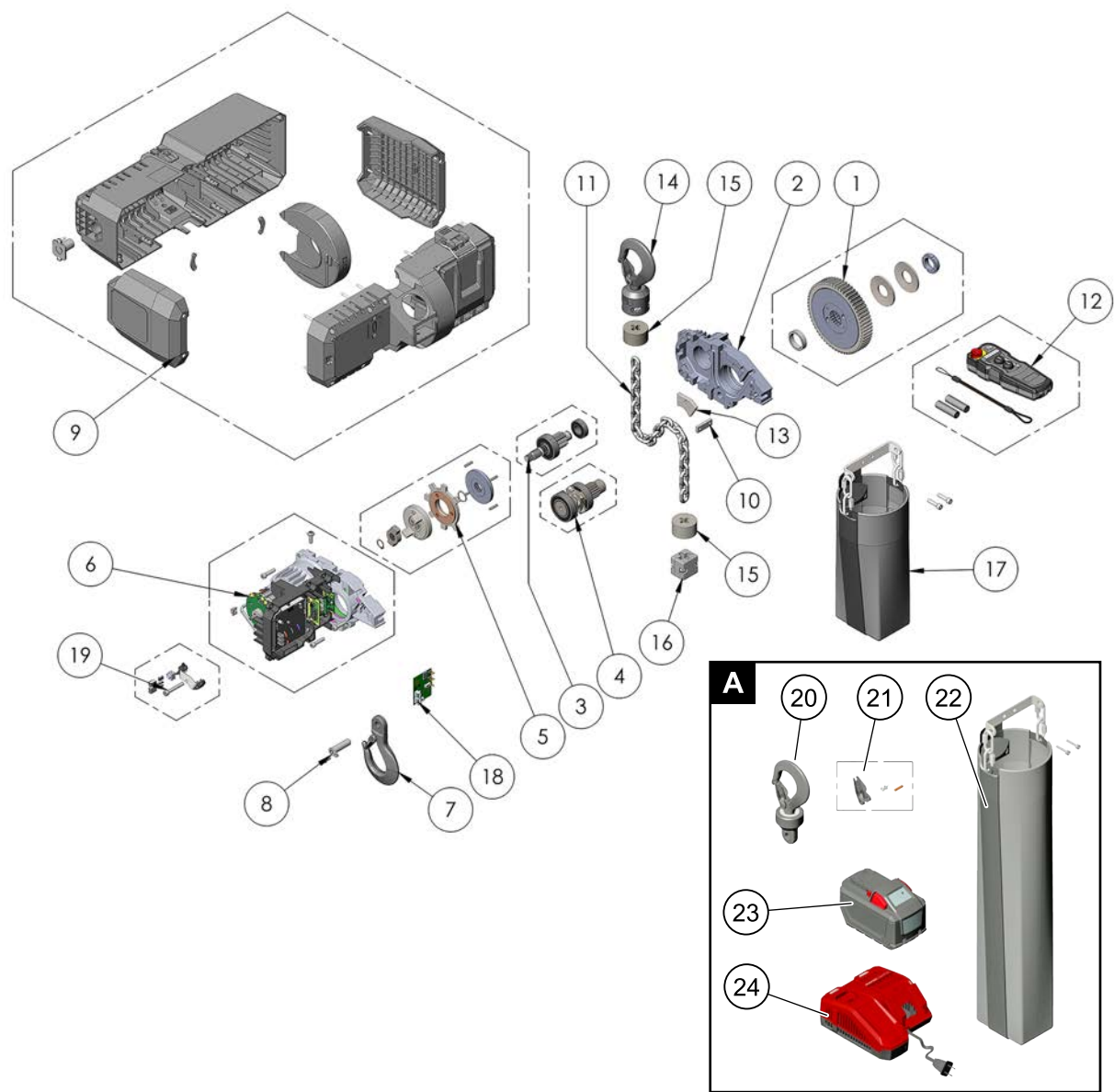
Figure 14. Pièces du palan
