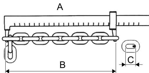
Figura 9. Medición del desgaste de la cadena
