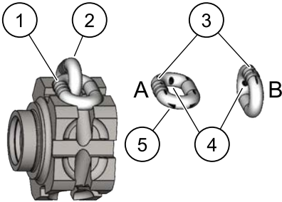
Figura 7. Áreas de desgaste da corrente
