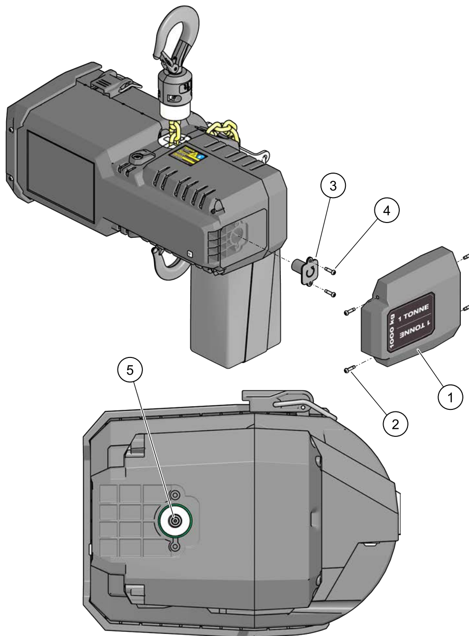
Figura 13. Procedimento de descida manual
